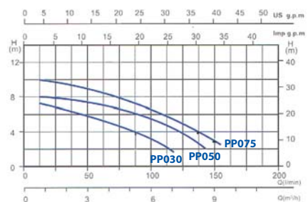
Curvas de rendimiento hidráulico Hydraulic performance curves Courbes de performances hydrauliques Curve delle prestazioni idrauliche
