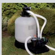
Depuradora arena (Caudal grupo 5 m 3 /h) Sand filter (Flow group 5 m 3 /h) Filtre à sable (Débit groupe 5 m 3 /h) Filtro a sabbia Portata gruppo 5 m 3 /h
