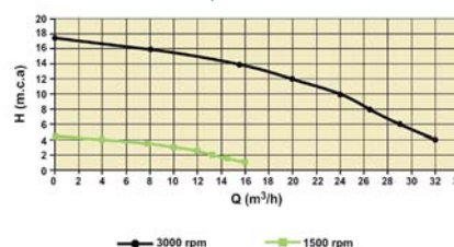
Curvas de rendimiento hidráulico Hydraulic performance curves Courbes de performances hydrauliques Curve delle prestazioni idrauliche
